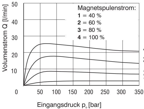
Nennvolumenstrom 15 l/min
