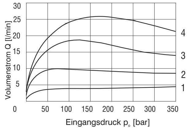
Nennvolumenstrom 8 l/min
