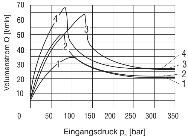
Nennvolumenstrom 15 l/min
