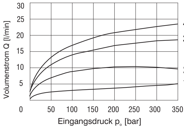
Nennvolumenstrom 5 l/min
