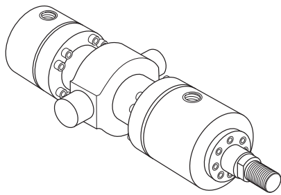
Befestigungsart MT4 Schwenkzapfen, mittig
